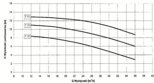
Charakterystyka pompy KS.7 KSM.7
