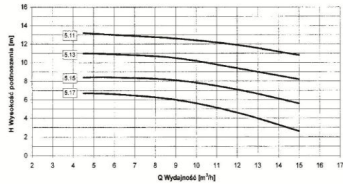
Charakterystyka pompy KS.5 KSM.5
