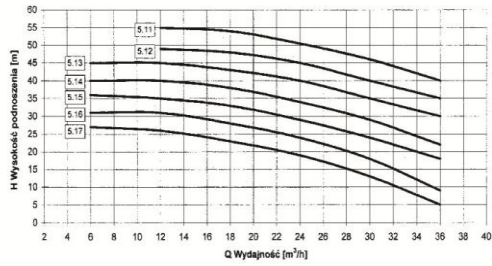
Charakterystyka pompy KS.5 KSM.5
