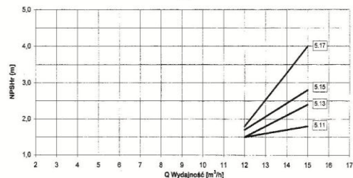
Charakterystyka pompy KS.7 KSM.7
