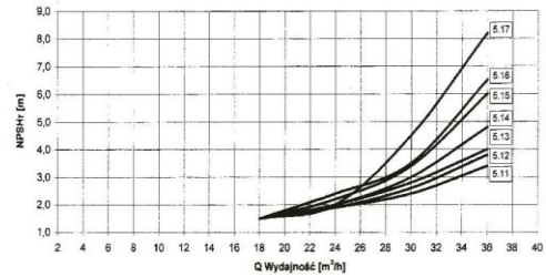
Charakterystyka pompy KS.7 KSM.7
