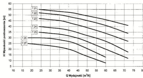
Charakterystyka pompy KS.7 KSM.7
