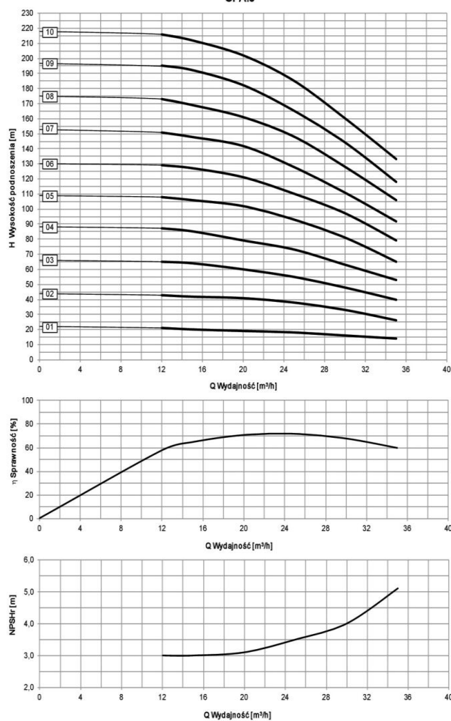
Charakterystyka pompy OPA.5
