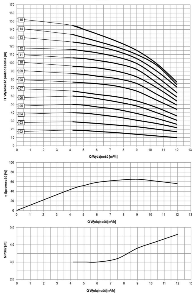
Charakterystyka pompy OPA.2
