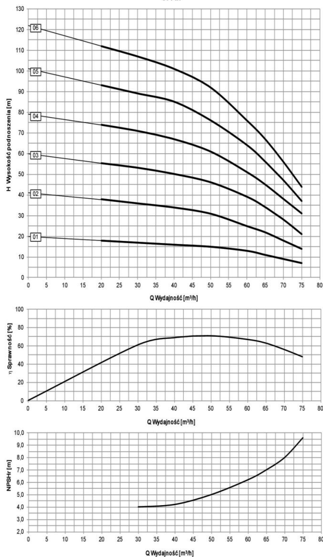
Charakterystyka pompy OPA.7
