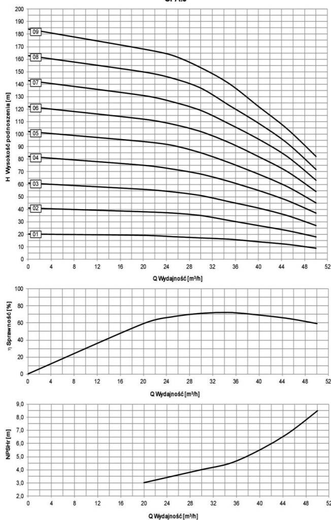
Charakterystyka pompy OPA.6
