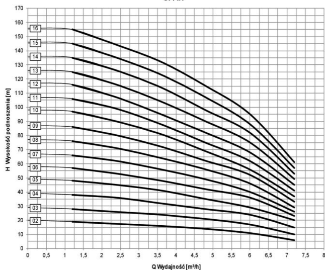
Charakterystyka pompy OPA.1
