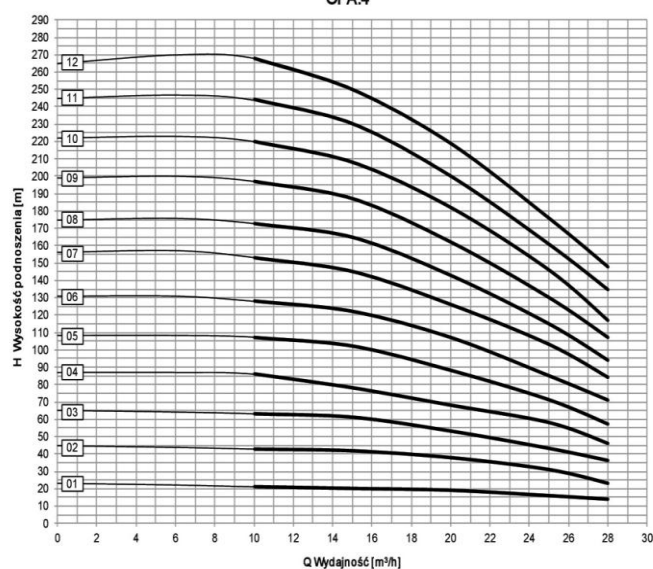
Charakterystyka pompy OPA.4
