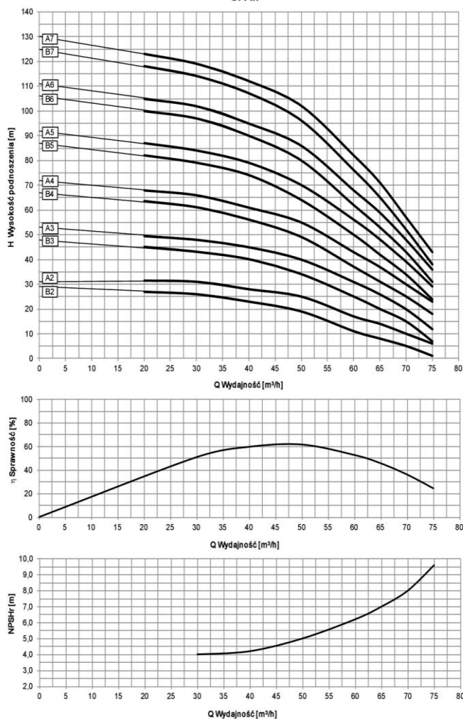
Charakterystyka pompy OPA.7
