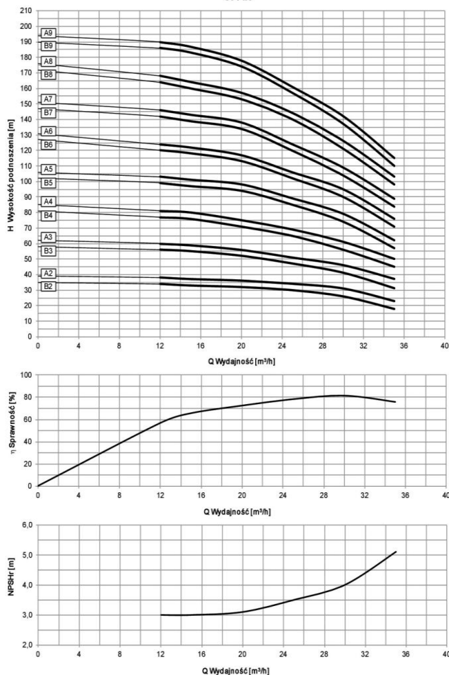
Charakterystyka pompy OPA.5
