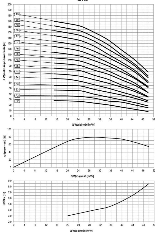
Charakterystyka pompy OPA.6
