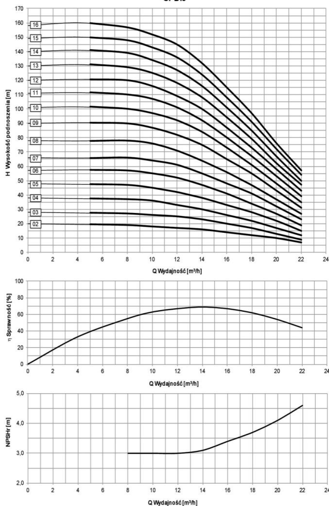
Charakterystyka pompy OPB.3
