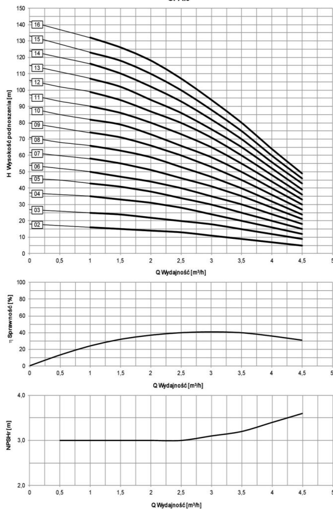
Charakterystyka pompy OPA.0
