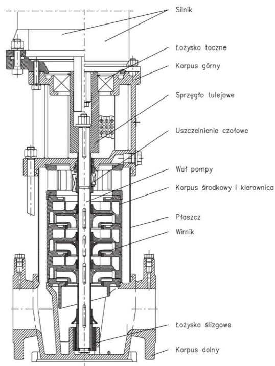
Przekrój pompy OPA.4 - OPA.7
