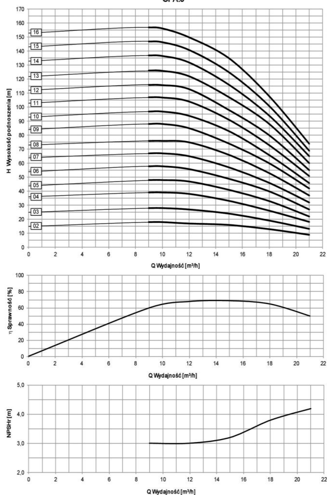
Charakterystyka pompy OPA.3
