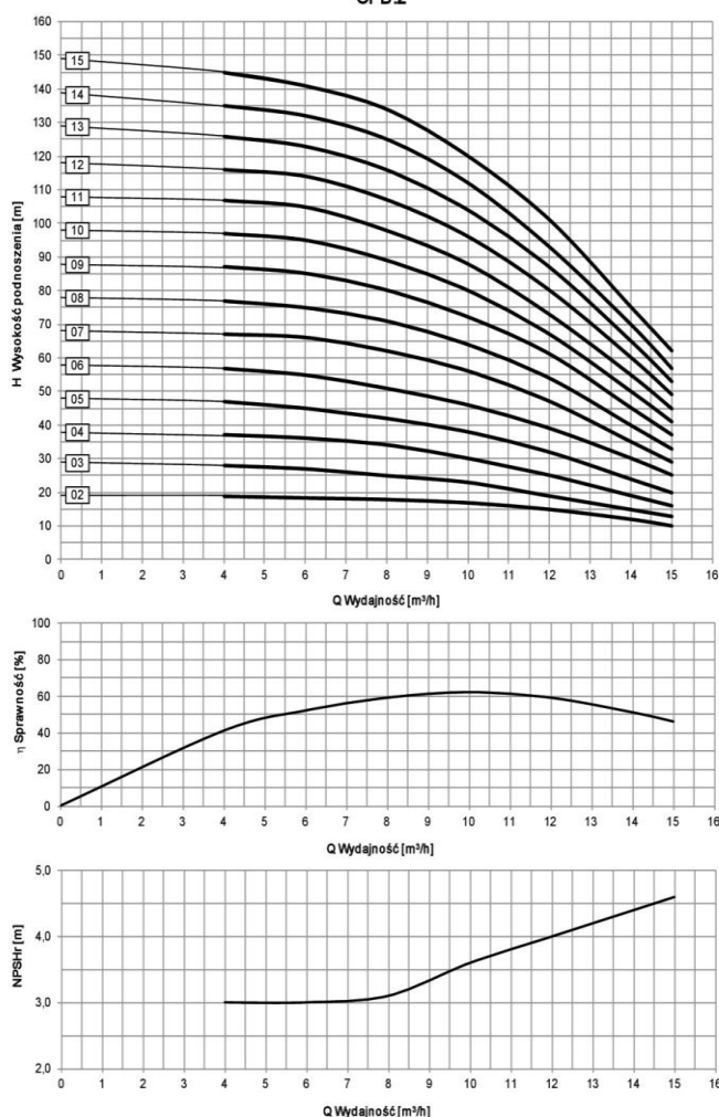
Charakterystyka pompy OPB.2
