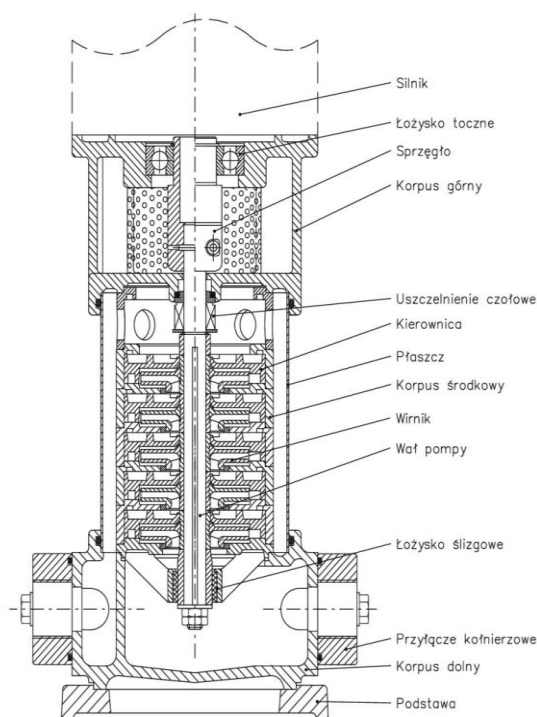
Przekrój pompy OPA.0 - OPA.3, OPB.2, OPB.3
