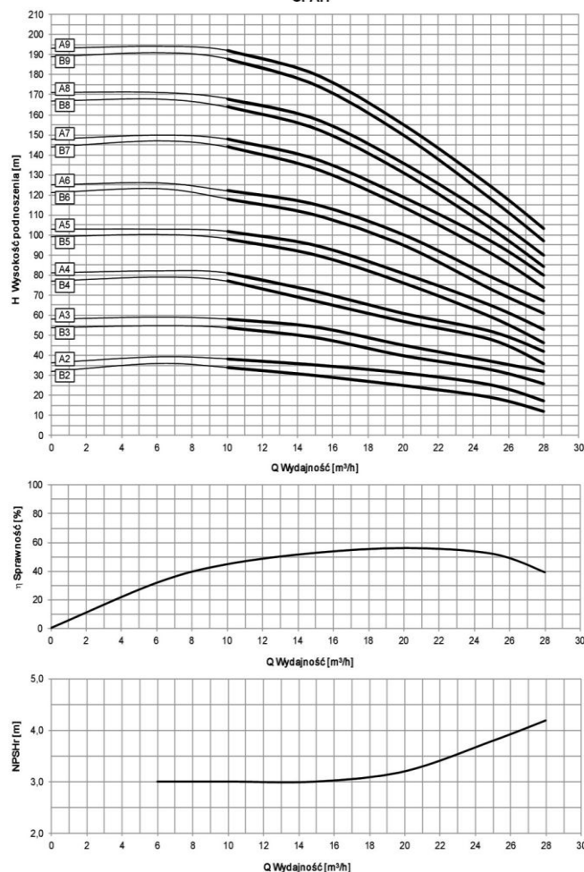
Charakterystyka pompy OPA.4
